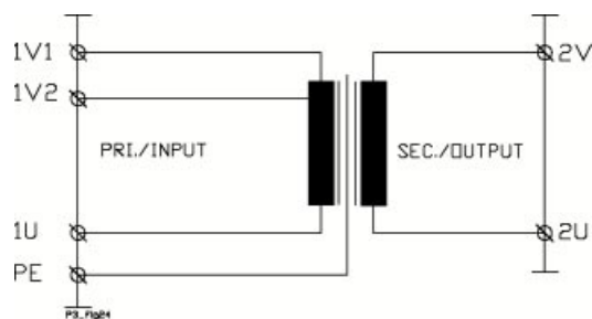
Pri. 400-415-440V
