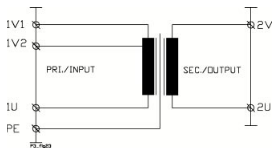
Pri. 230-250V
